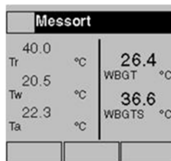
Obr. 4 - Ukážka displeja meracieho prístroja.
