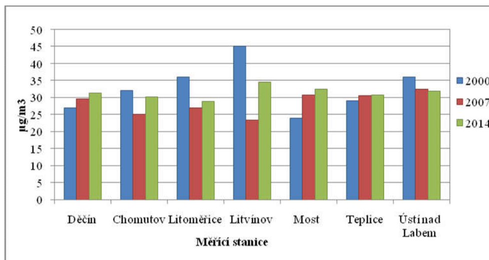
Obr. 4 - Průměrné roční koncentrace \text{PM}_{10} v \mu\text{g}/\text{m}^3 v Ústeckém kraji v letech 2000, 2007, 2014 [6]
